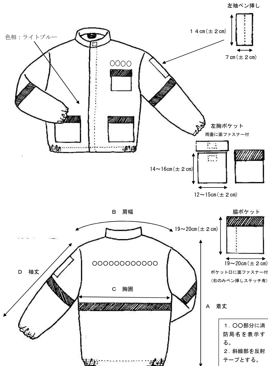
別図1 感染防止衣（上衣）の形状及び寸法
