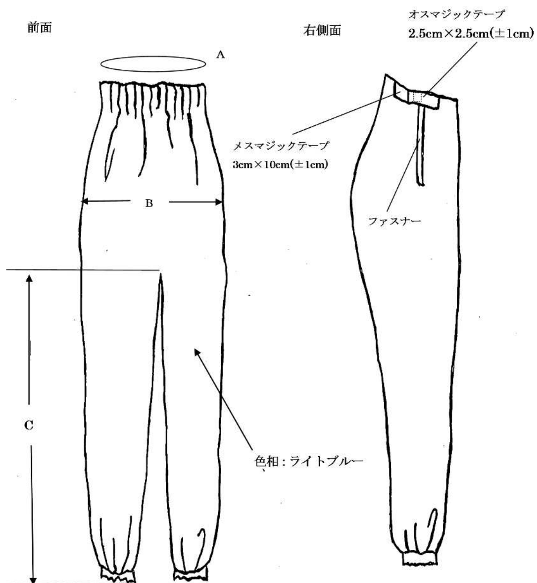
別図2 感染防止衣（下衣）の形状及び寸法
