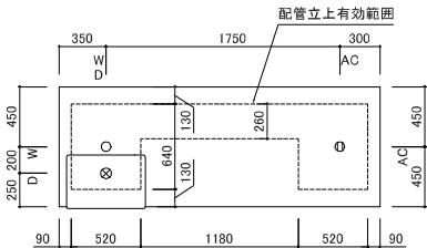
配管立上り図 S=1/30
