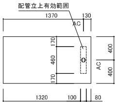
配管立上り図 S=1/30
