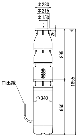
寸法図
