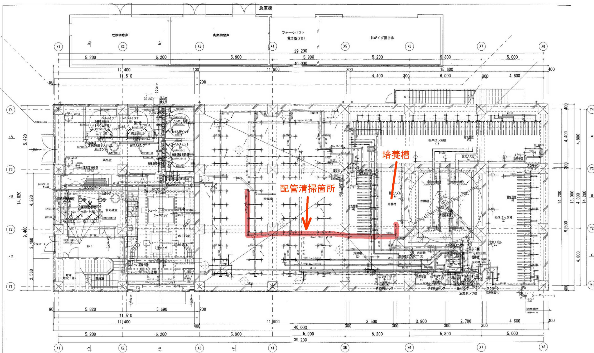
1階平面図 S=1/60
