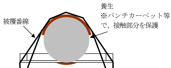
径の大きな支柱の場合
