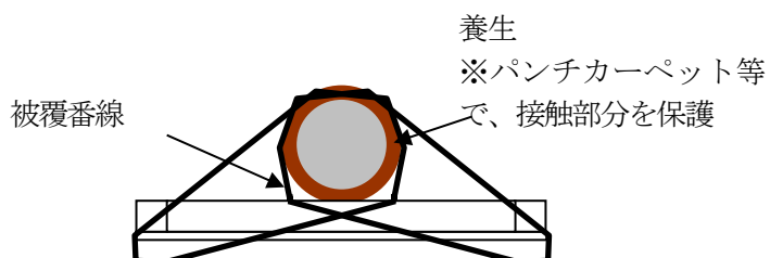
径の大きな支柱の場合
