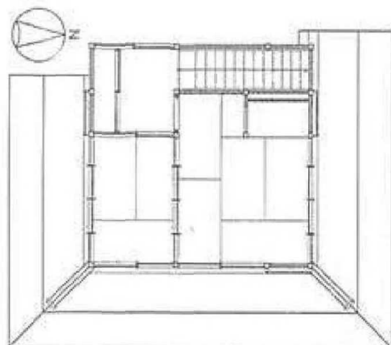
2階平面図
