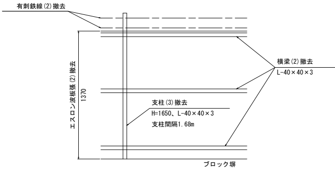
正面図
