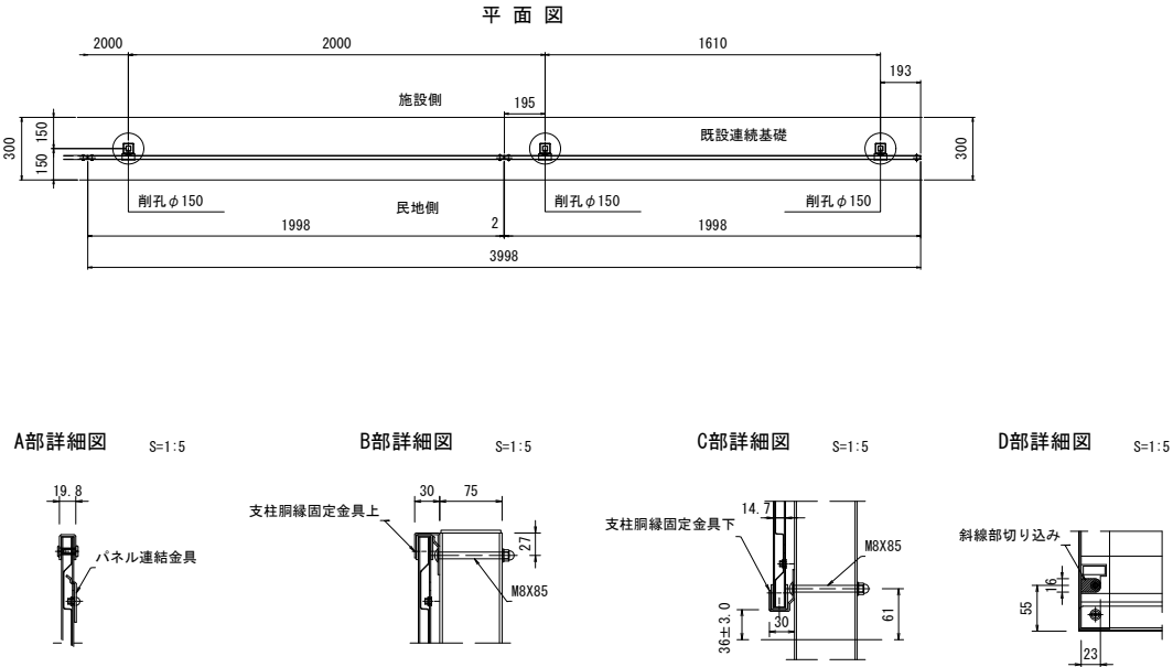
目隠しフェンス(2) H=1.2m S=1:20
