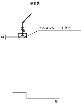
笠木コンクリート撤去
