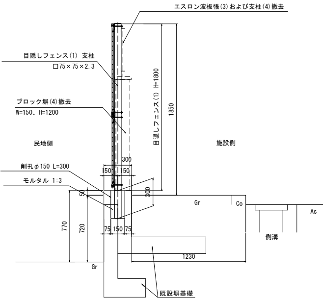
標準断面図4-4 フェンス基礎(1)削孔
