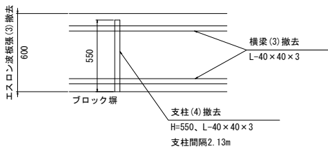
正面図
