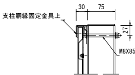
B部詳細図 S=1:5
