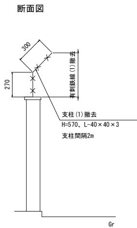
有刺鉄線(1)撤去 支柱(1)撤去
