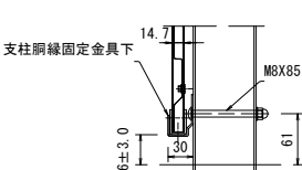
C部詳細図 S=1:5
