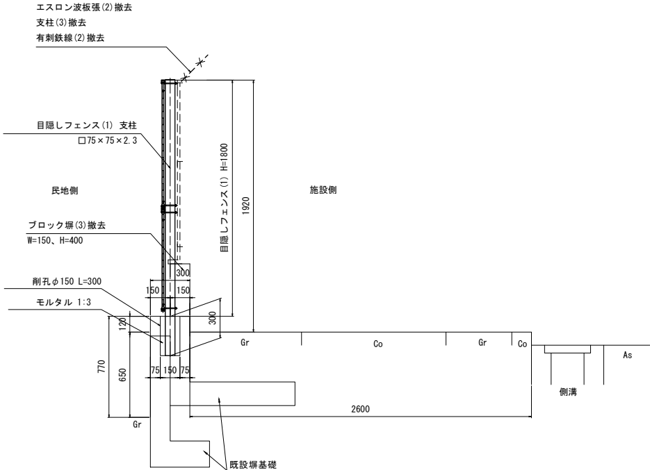
標準断面図3-3 フェンス基礎(1)削孔
