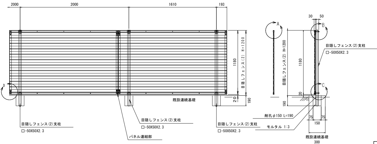
正面図
