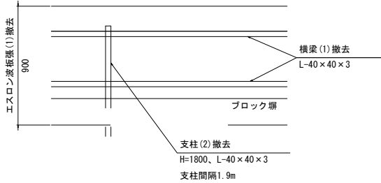
正面図
