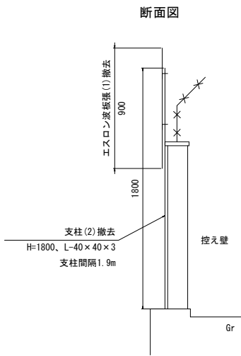
エスロン波板張(1)撤去 支柱(2)撤去 横梁(1)撤去
