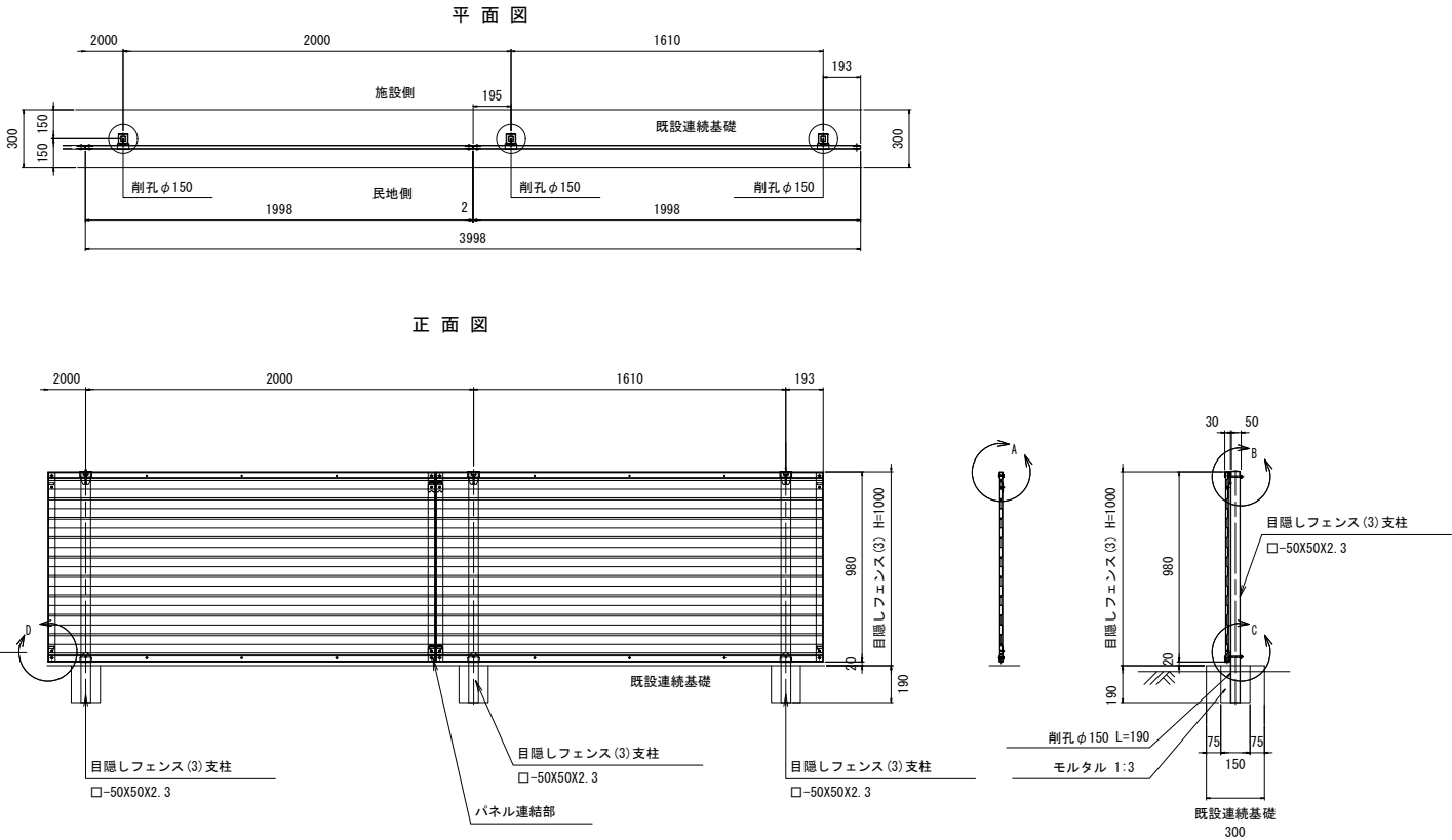
目隠しフェンス(3) H=1.0m S=1:20
