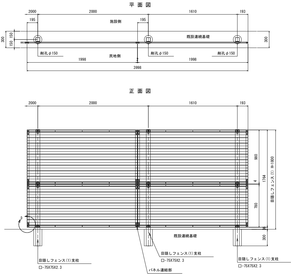
目隠しフェンス(1) H=1.8m S=1:20
