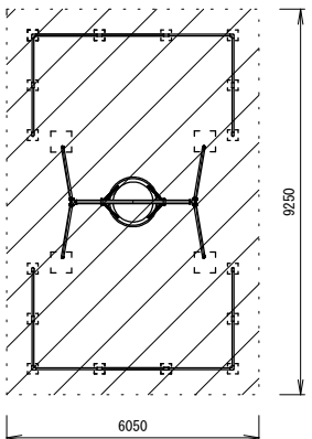
吊席詳細図 S=1/40
