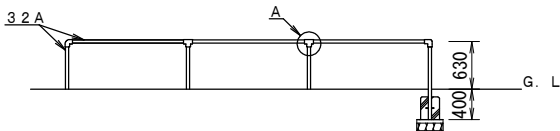
境界柵正面図 S=1/100
