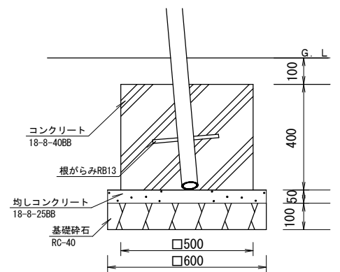
ブランコ基礎詳細図 S=1/20
