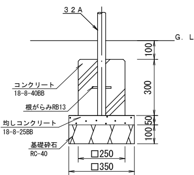
境界柵基礎詳細図 S=1/20
