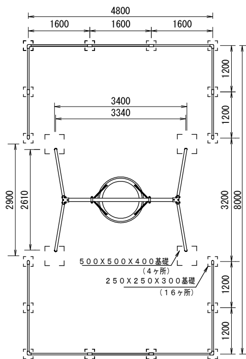
平面図 S=1/100
