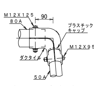
C詳細図 S=1/12
