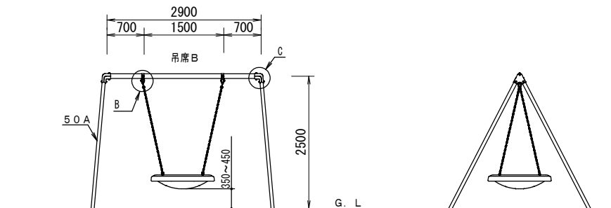
正面図 S=1/100
