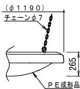
吊席詳細図 S=1/40
