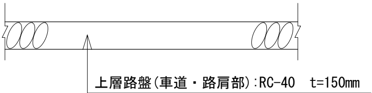
碎石舗装 S=1:20
