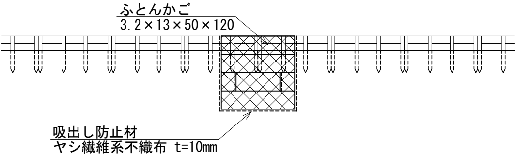
正面図 S=1:100
