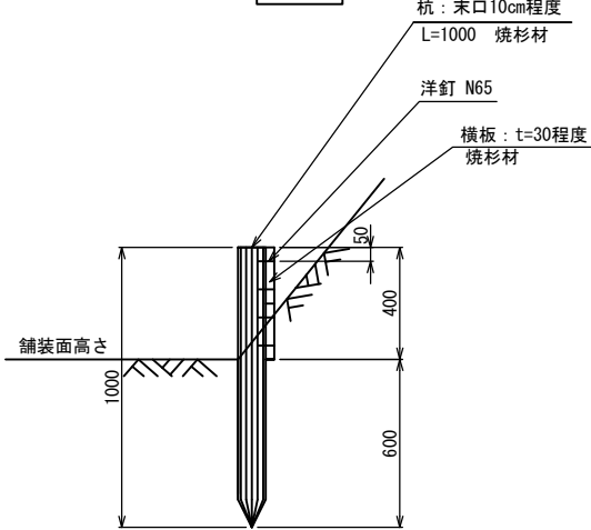
断面図
