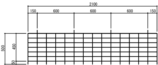
獣害防止用メッシュパネル スカート部
