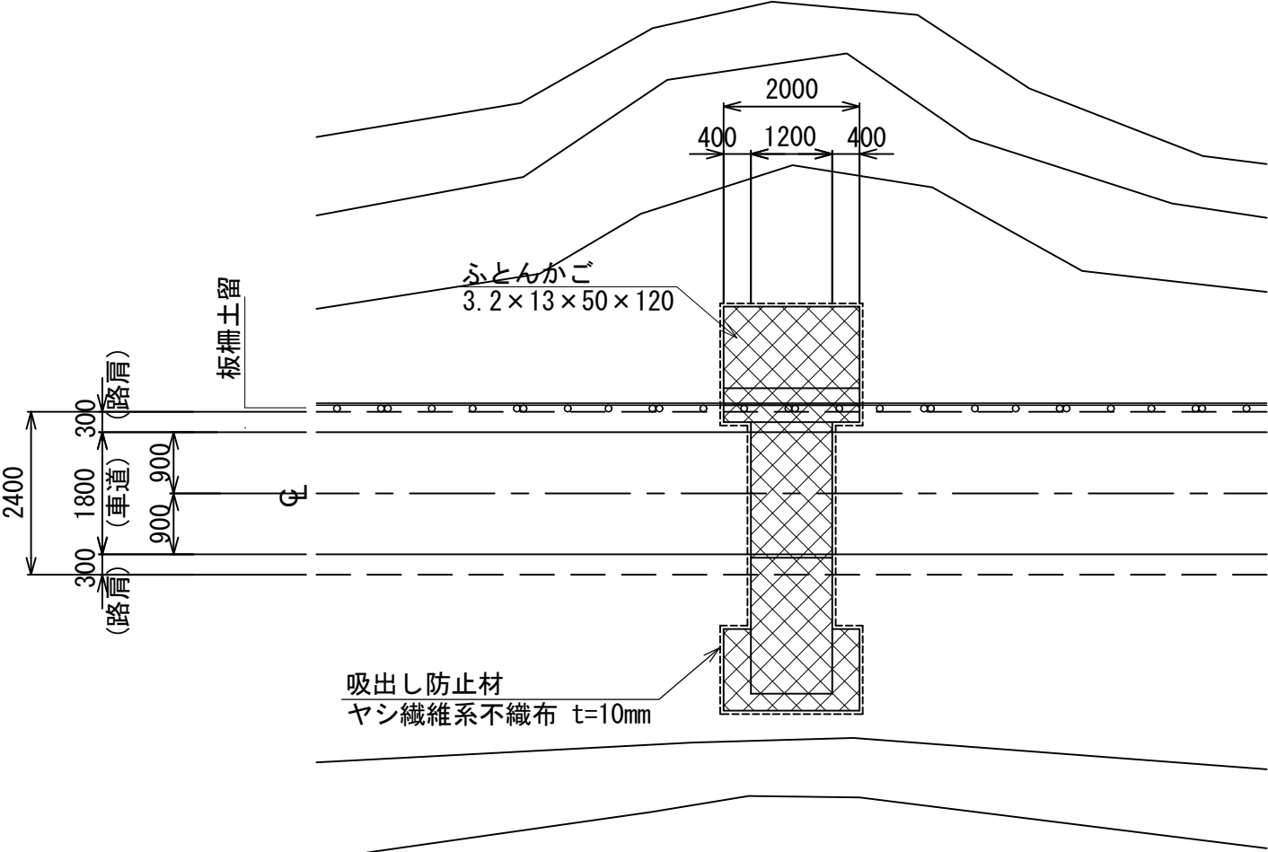
正面図 S=1:100
