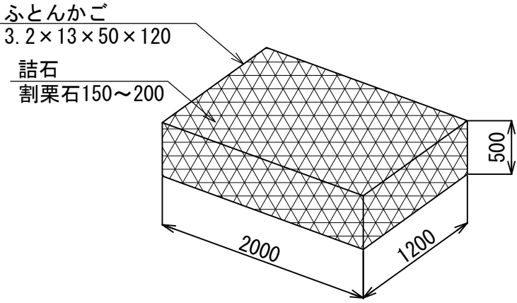
ふとんかご詳細図 S=1:50
