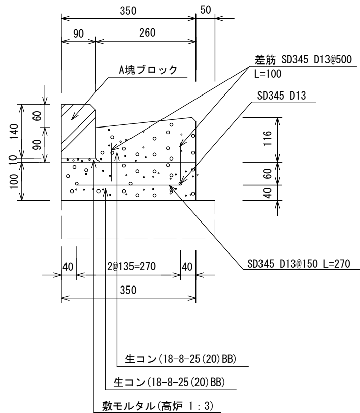
A-A断面図
