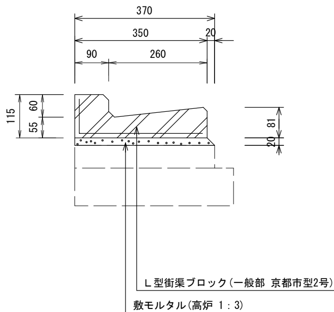
A-A断面図
