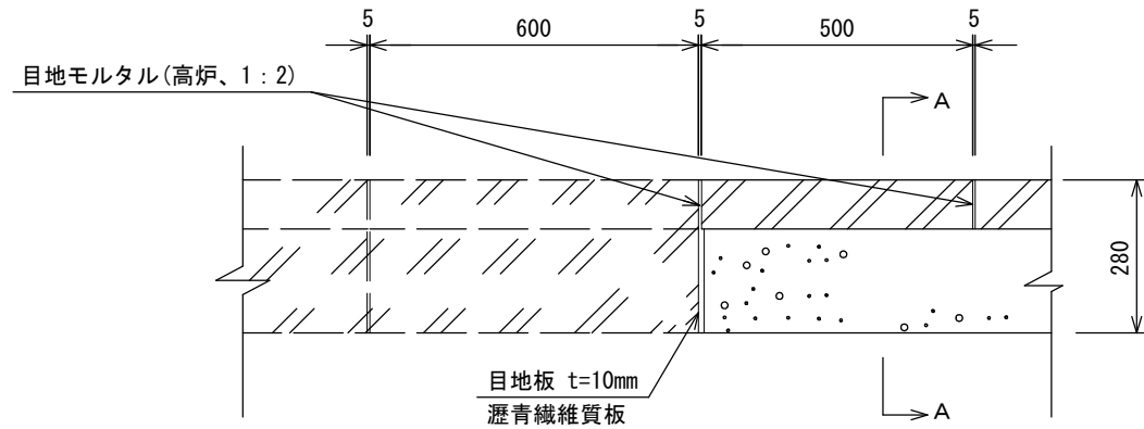
平面図
