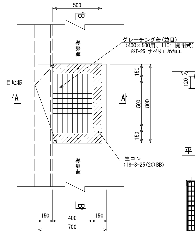
平面図
