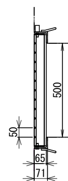
断面図
