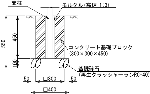
A-A断面図
