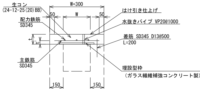
断面図
