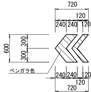
矢羽根（生活道路） S=1/50
