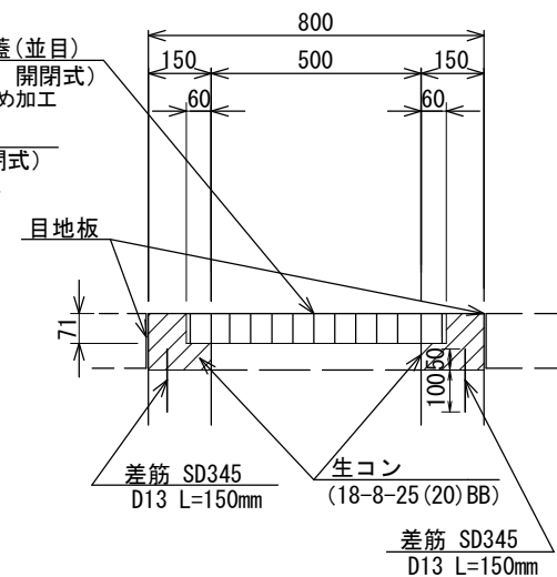
断面図
