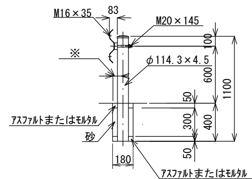
断面図 S=1/40
