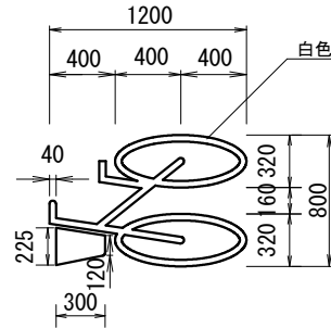
自転車マーク（幹線道路） S=1/50
