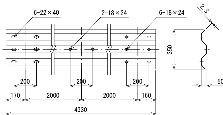
ビーム S=1/20
