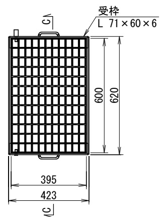
平面図
