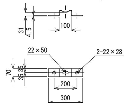
ブラケット S=1/20
