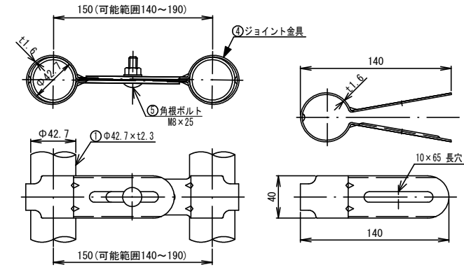
ジョイント金具詳細図 (1/5)
