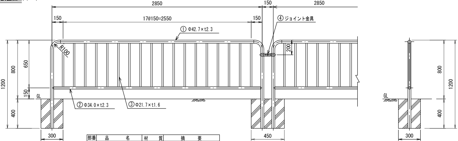
設置図 (1/25)
