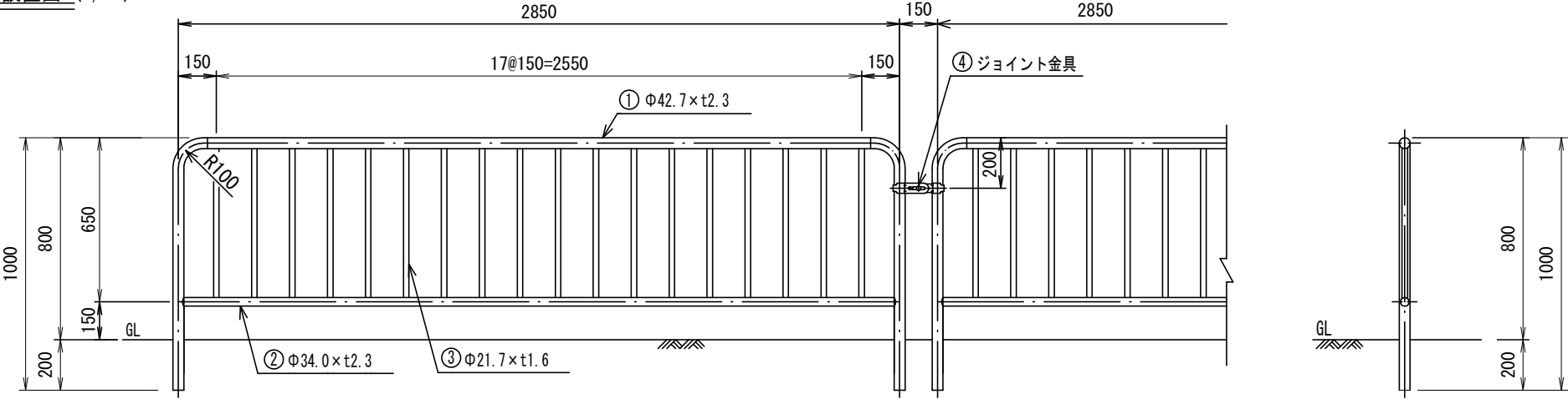
設置図 (1/25)
