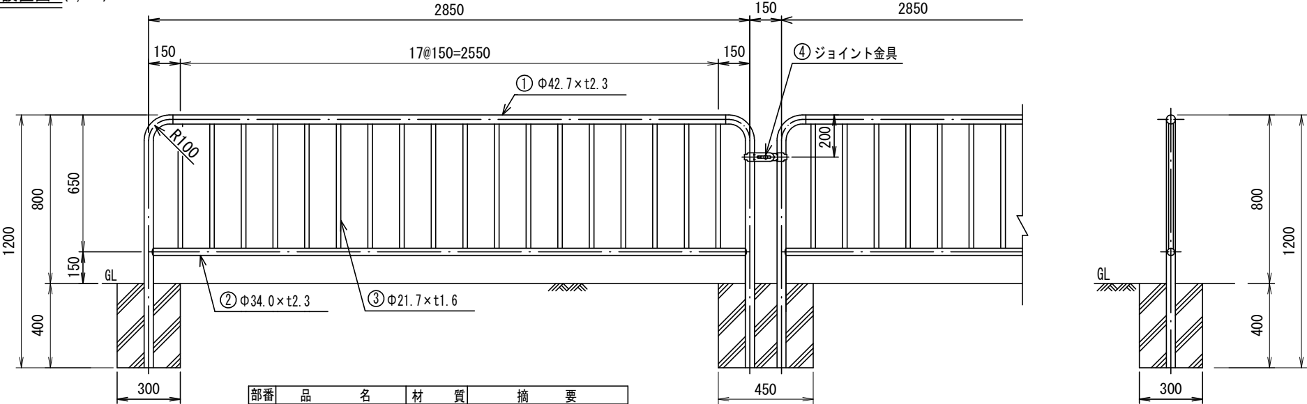
設置図 (1/25)
