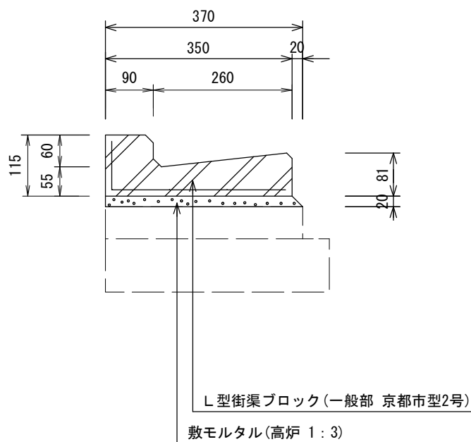
A-A断面図
