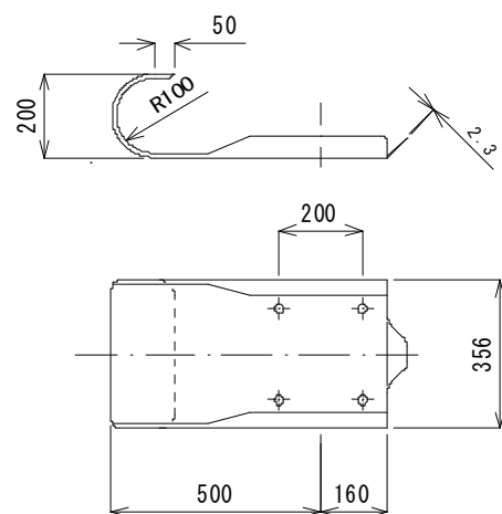
袖ビーム
