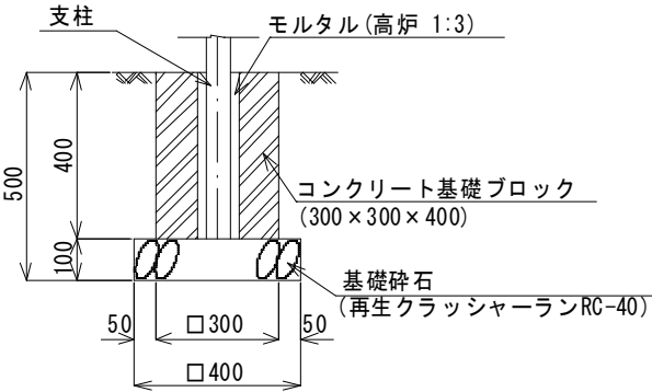
A-A断面図
