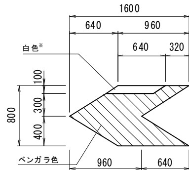
矢羽根(幹線道路) S=1/50
