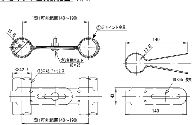
ジョイント金具詳細図 (1/5)
