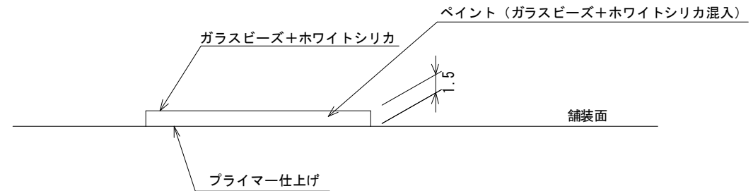
断面図
