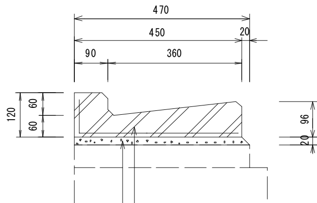
A-A断面図
