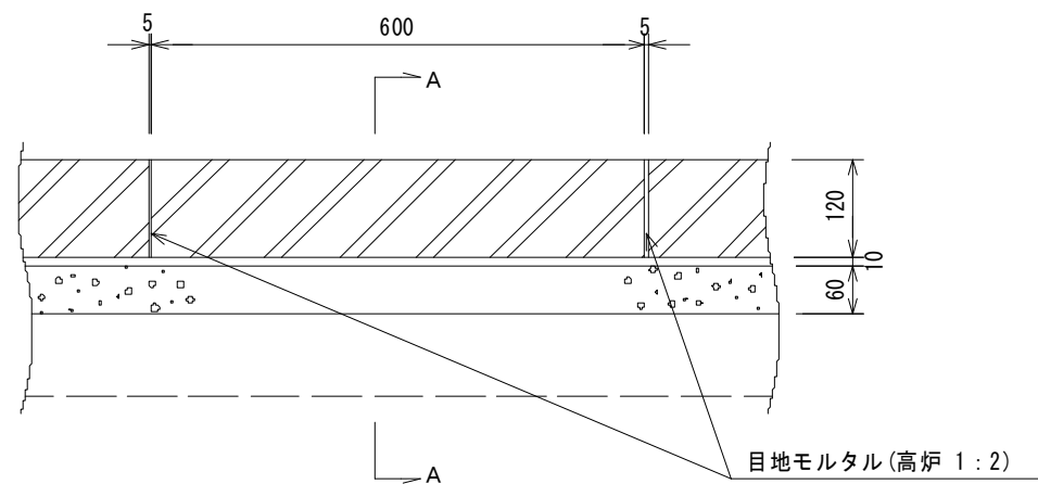
側面図
