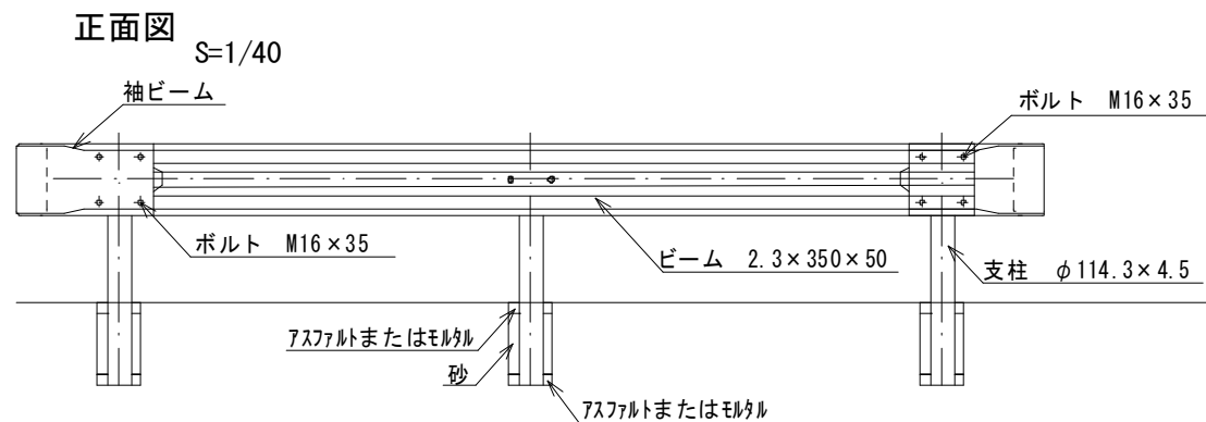
袖ビーム
