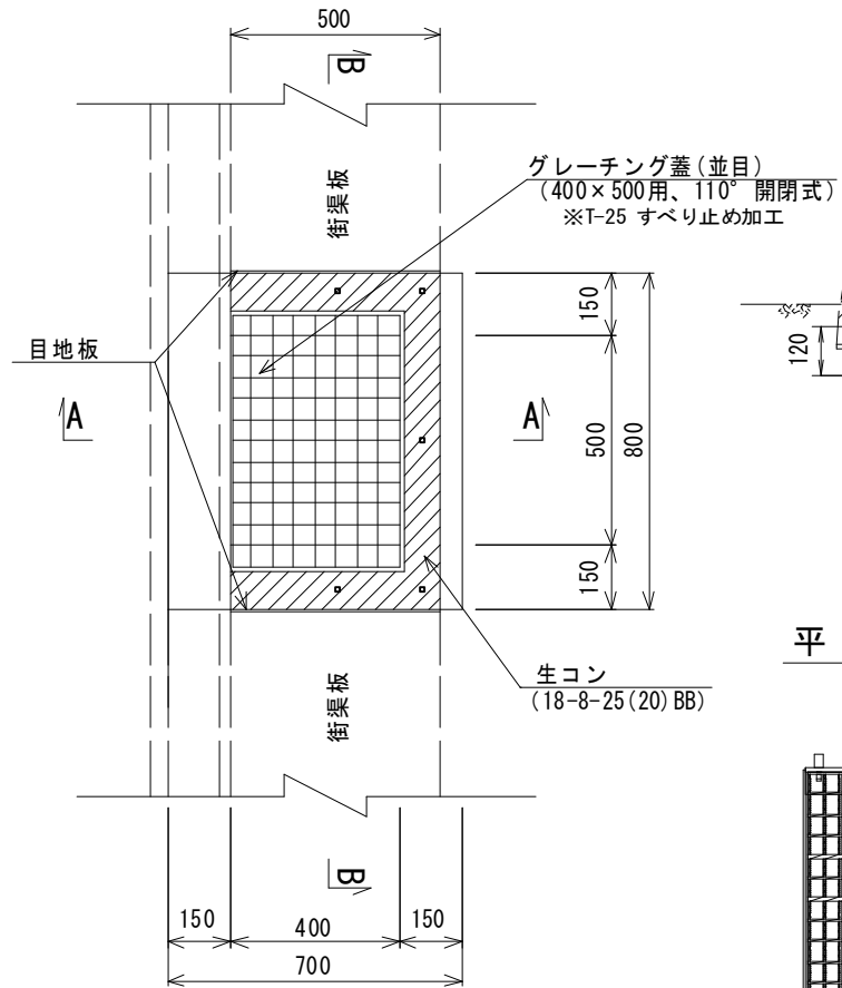
平面図
