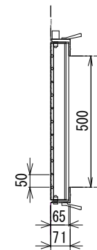
断面図 C-C
