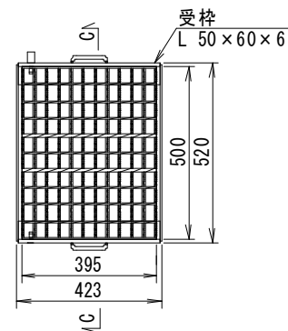
平面图
