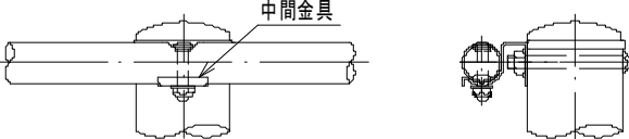
中間部詳細図 (1/10)
