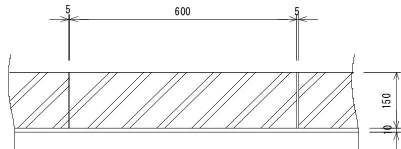
側面図
