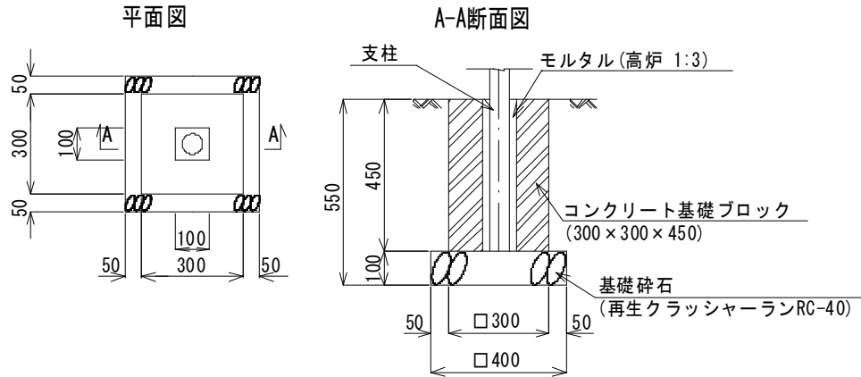
横断防止柵基礎ブロック詳細図 (1/20)
