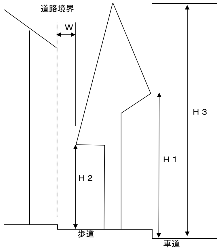
縦断標準断面
