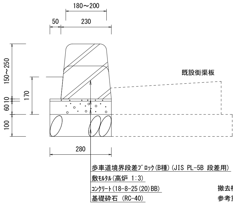
段差部 S=1:10
