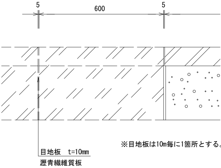
平面図 S=1:20
