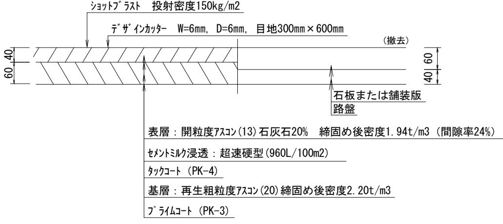
特殊ブロック舗装 視覚障害者誘導用標示 S=1:10
