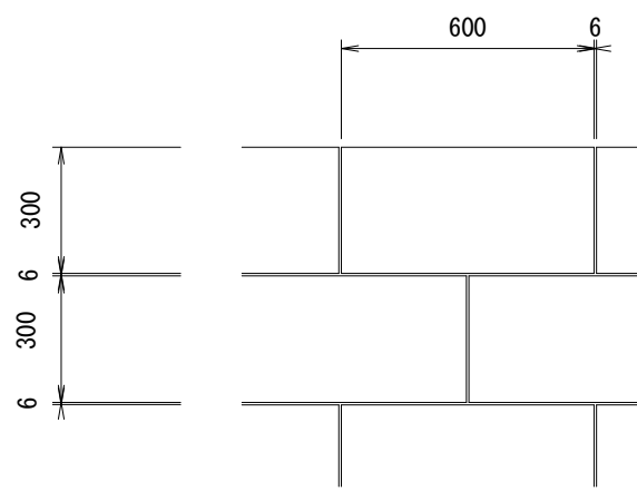
デザインカッター（パターン図） S=1:20
