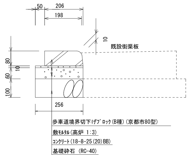
横断部 S=1:10
