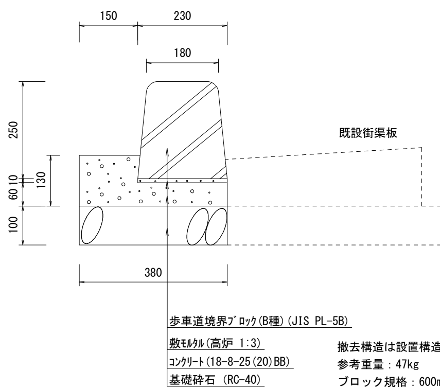
一般部 S=1:10
