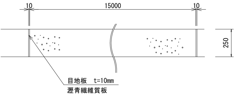
平面図 S=1:20
