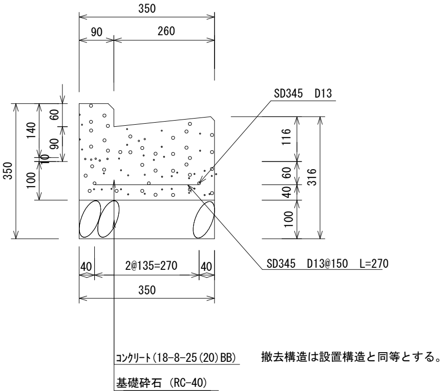
現場打L型側溝 S=1:10
