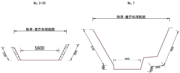
第1工区(三宝寺川) S=1/200
