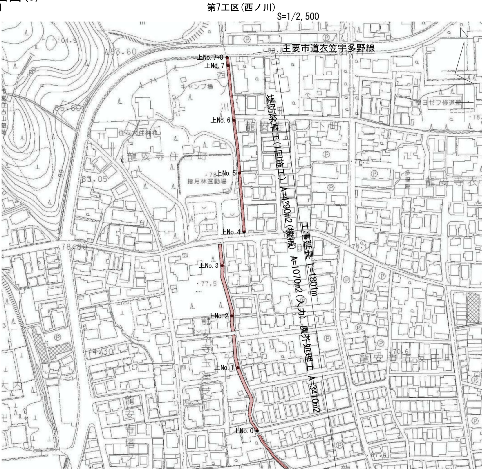
平面図・断面図(5) 西ノ川
