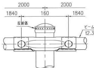
取付部詳細図 (1/4)
