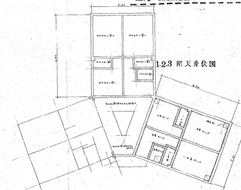
1.2.3 階天井伏図
