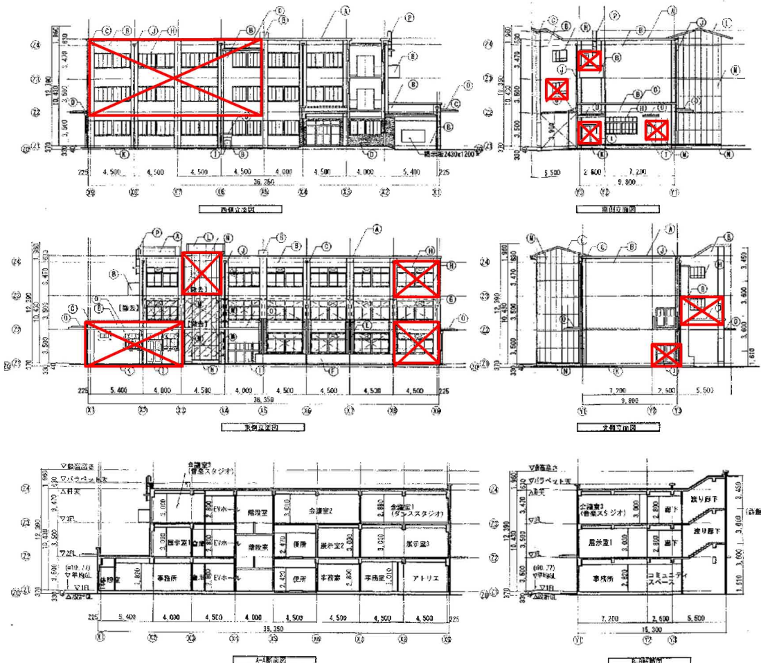
本館立面図
