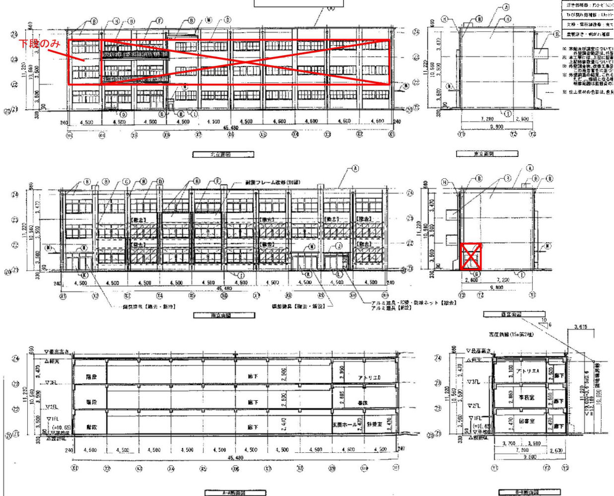
北館立面図
