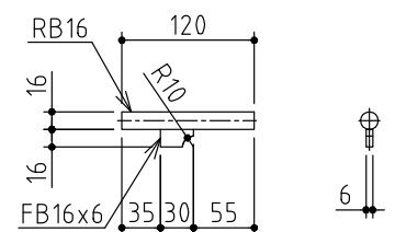
ロックピン詳細図 ※スチール製
