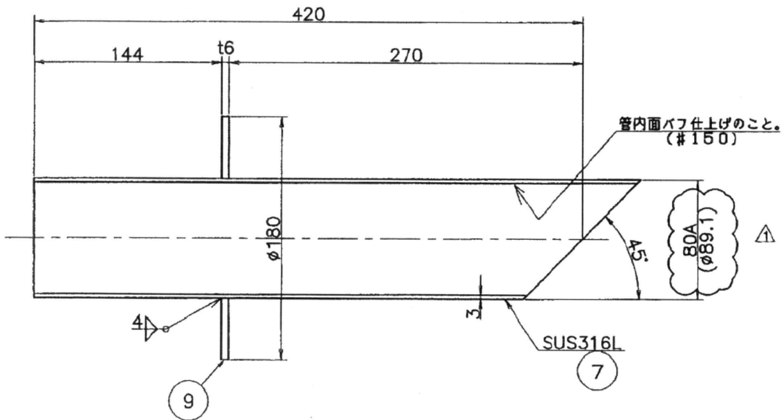
薬剤噴射ノズル詳細
