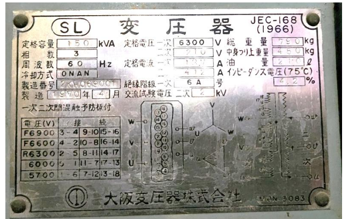
変圧器 (銘板)
