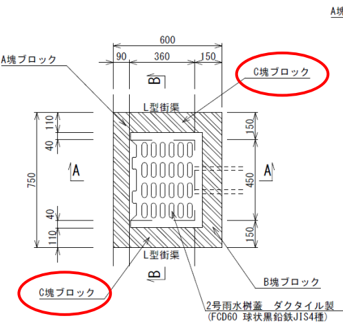
平面図 S=1/20
