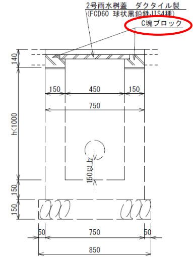
B-B断面 S=1/20
