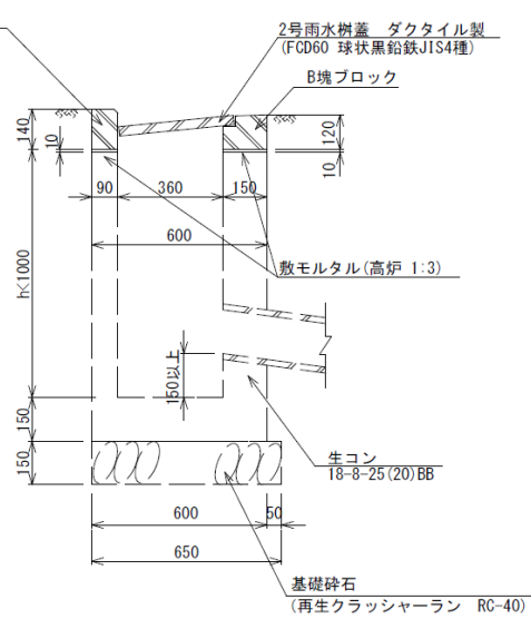
A-A断面 S=1/20
