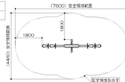
安全領域範圍 S= 1 : 100
