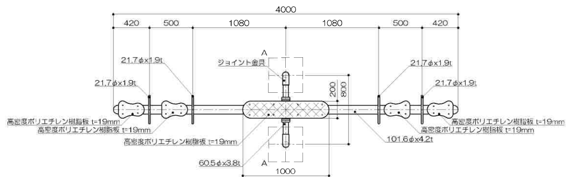
平面図 S= 1 : 30
