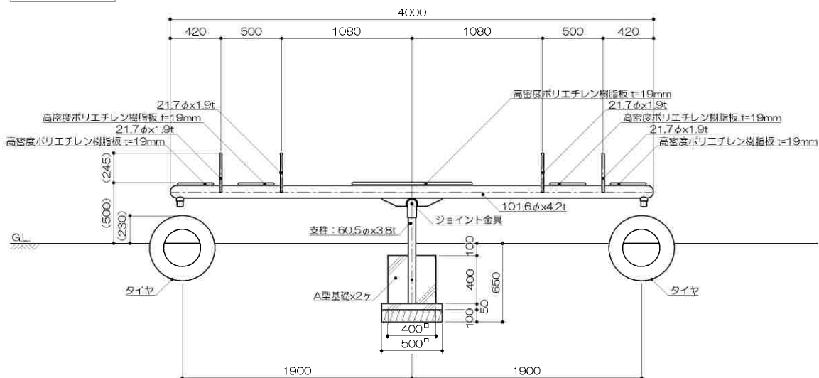
立面图 S=1:30
