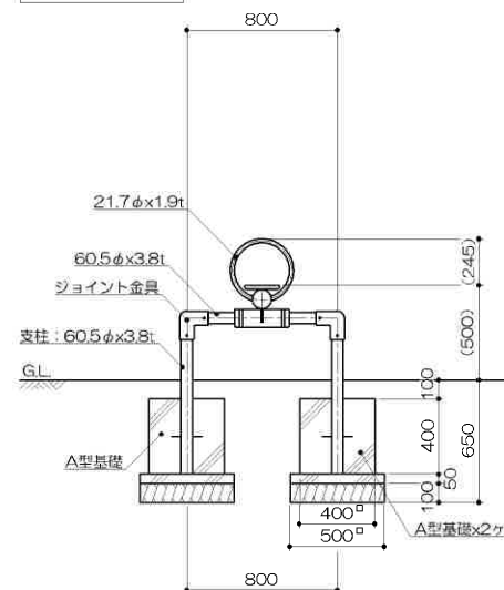
側面図 S= 1 : 30
