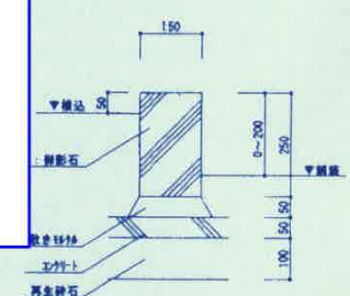
石縁石詳細図 1:10(A1)
