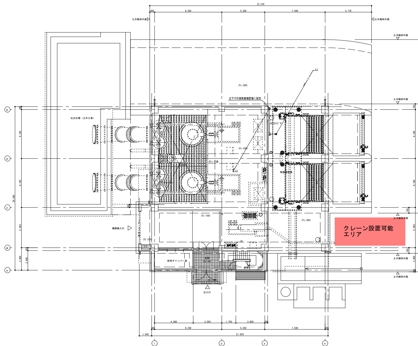
1 階平面図 1/100
