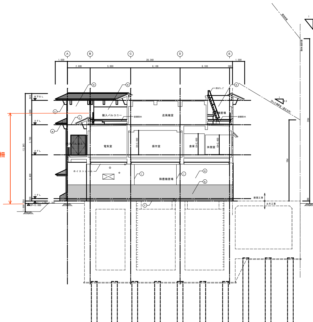
断面図 d
