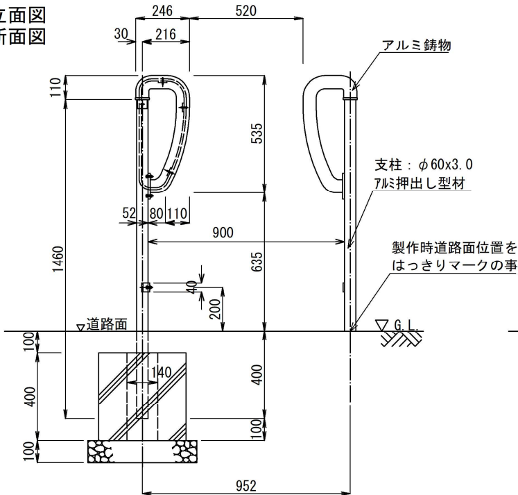
側面図 断面図
