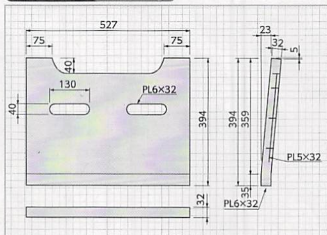
コンクリート蓋 参考重量:29kg
