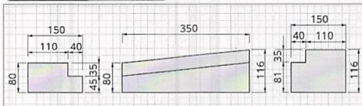
C 塊 参考重量:12kg
