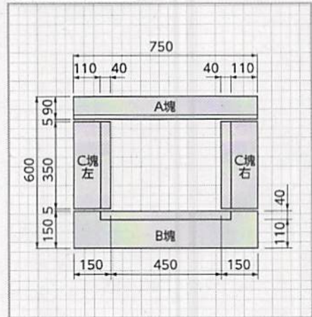
緑塊組立平面図
