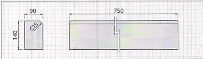
A塊乗入れ用 参考重量:16kg
