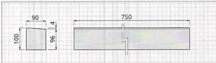
B 塊 参考重量:30kg
