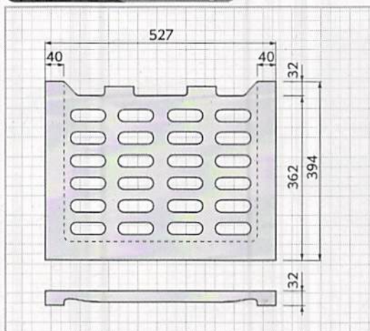
ダクトイル蓋 参考重量:29kg
