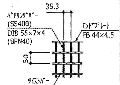
グレーチング構造図
