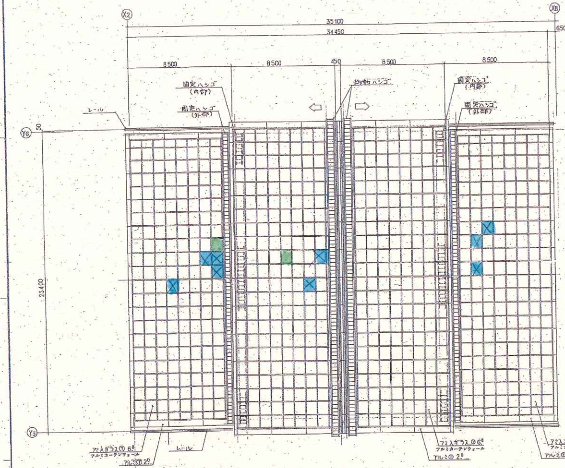
屋根伏図 SCALE 1:100
