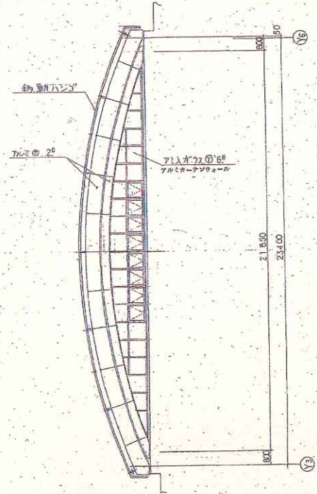
立面図 SCALE 1:100
