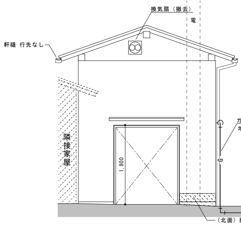
北立面図 (1/50(A3))
