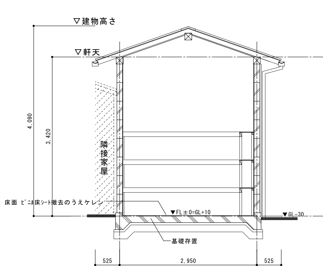
断面図 (1/50(A3))
