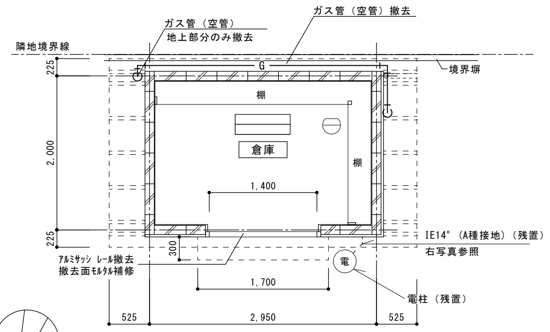
平面図 (1/50(A3))
