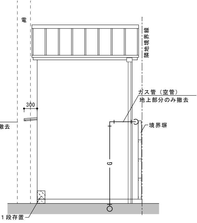
西立面図 (1/50(A3))
