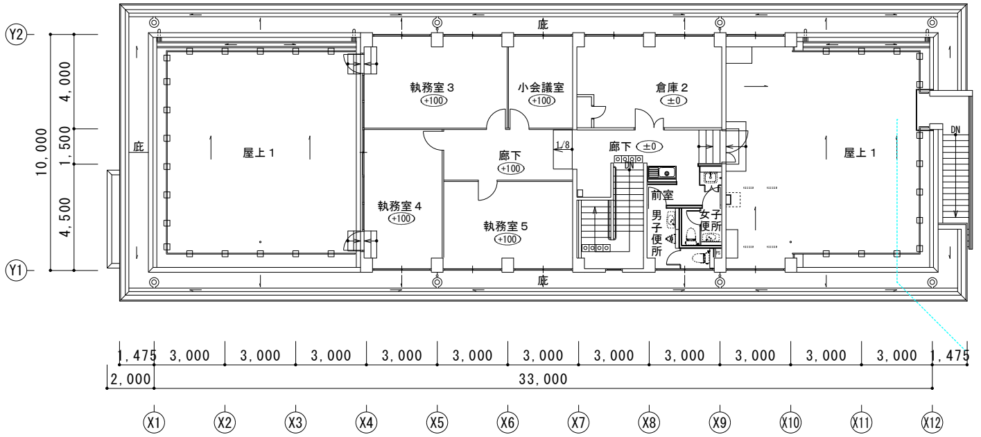
京都市監査事務局 2階平面図
