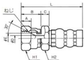
管用平行めねじ (めすシート)
