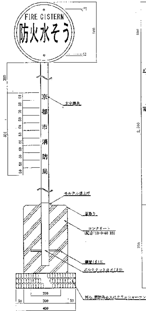
(正面図)
