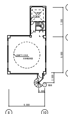
5 階平面図 NO SCALE
