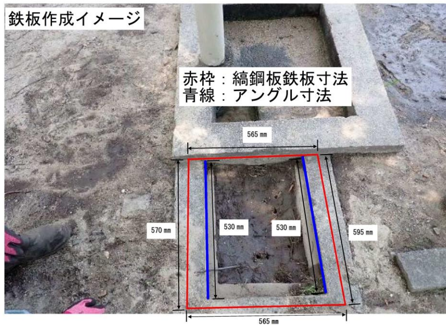
アングル溶接位置イメージ
