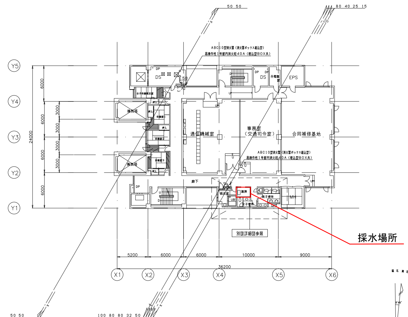
3階平面図 1:400
