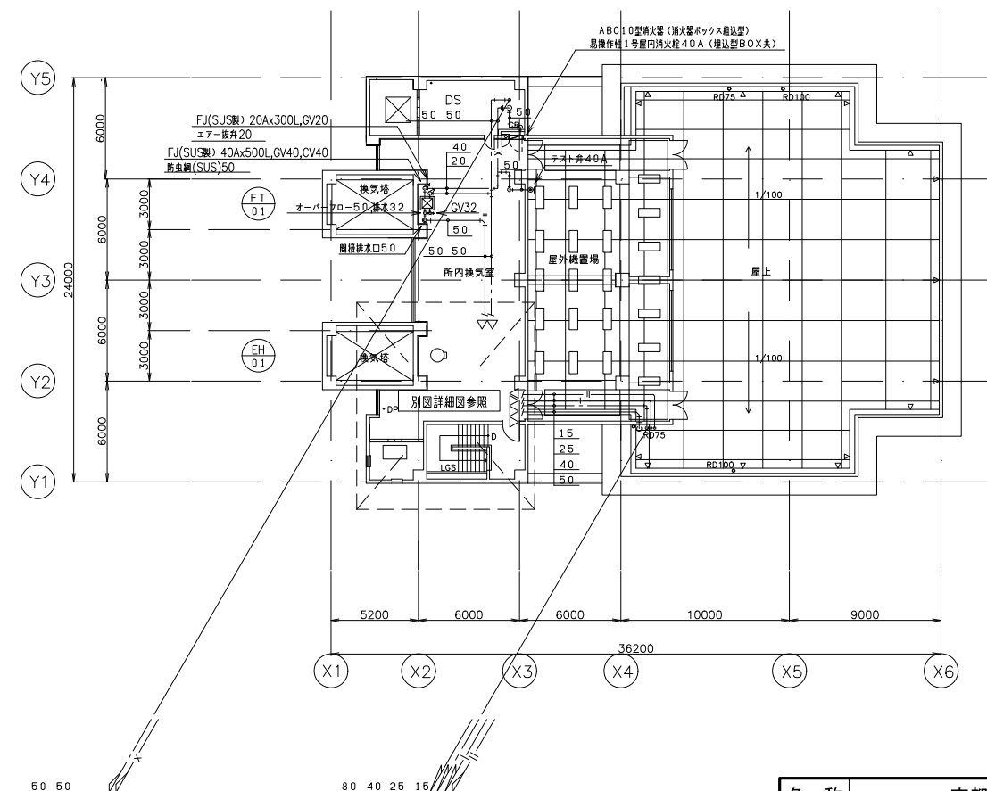
4階平面図 1:400
