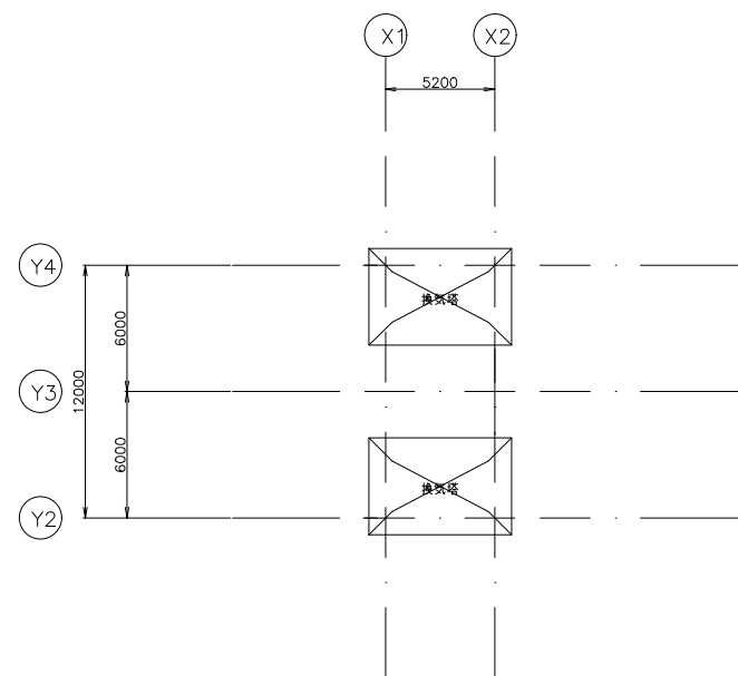
換気塔屋根伏図 1:400
