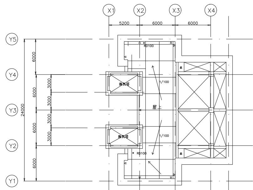
R階平面図 1:400
