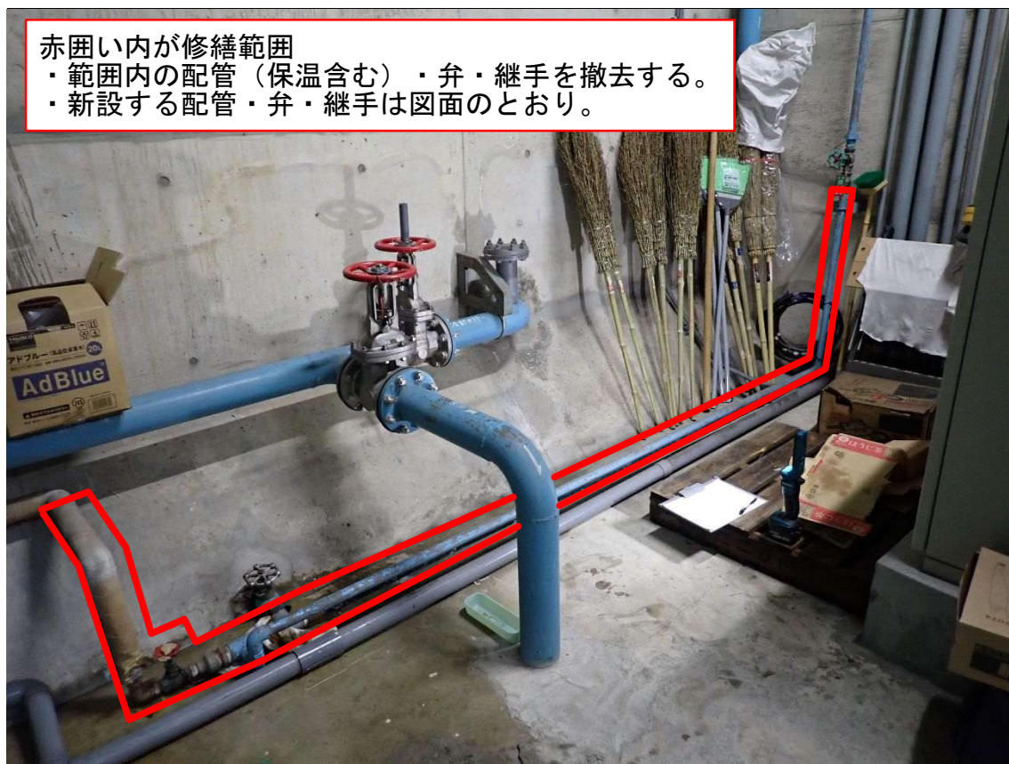
現状写真 1
