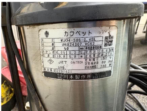
写真8：支給品ポンプ銘板
