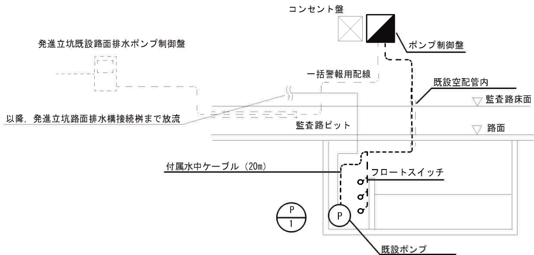
修繕系統図 N. S.
