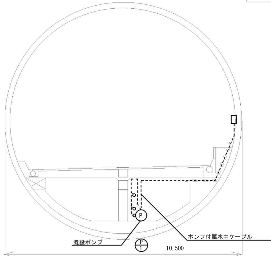
A-A' 断面図 N. S.
