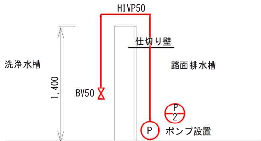
P-2 配管イメージ図N. S.
