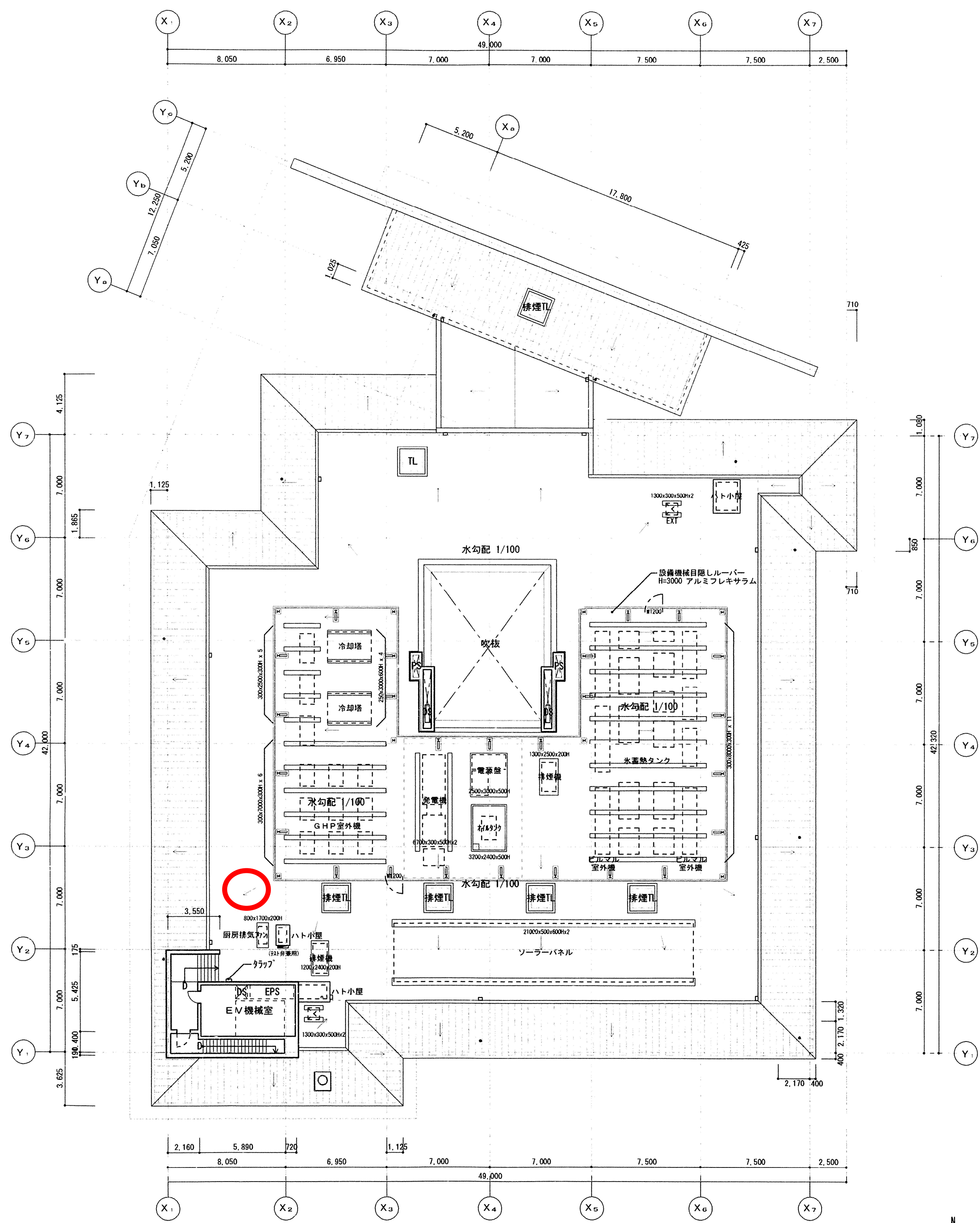
屋根平面図 (屋上平面図)
