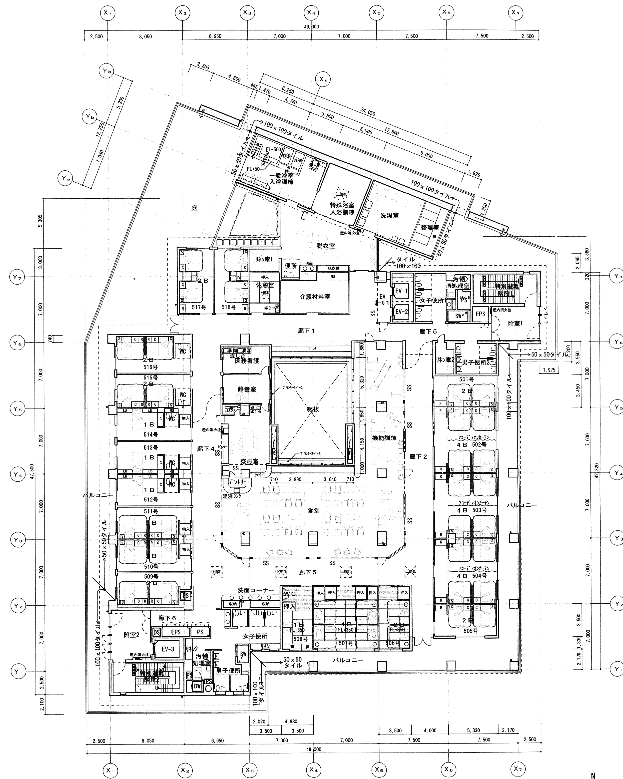
5 階 平 面 図
