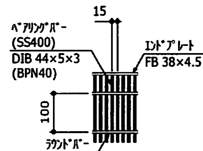
グレーチング構造図
