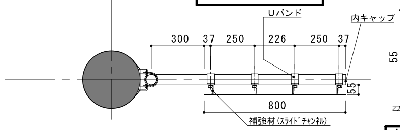
歩道用平面図
