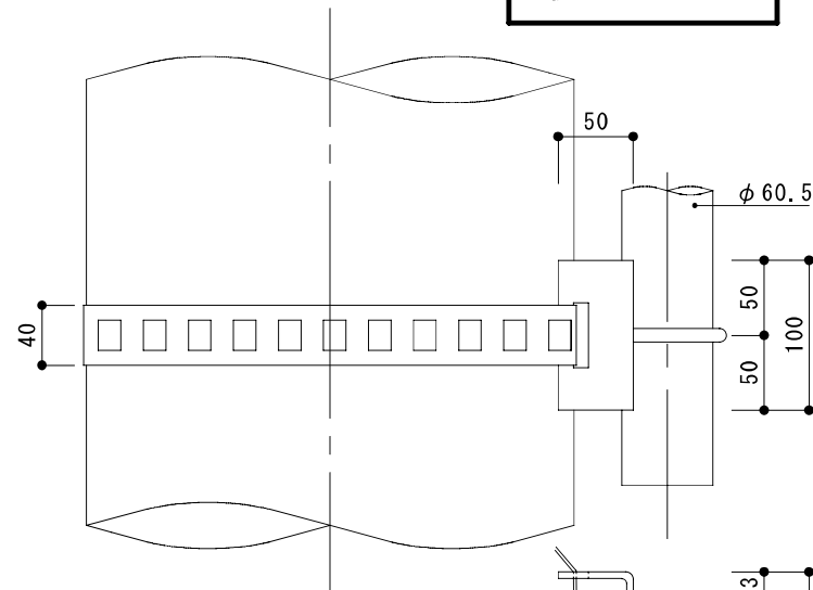
側面図
