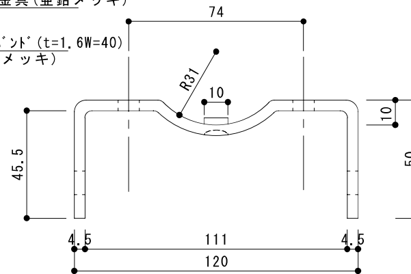
誘導標識標準図－2
