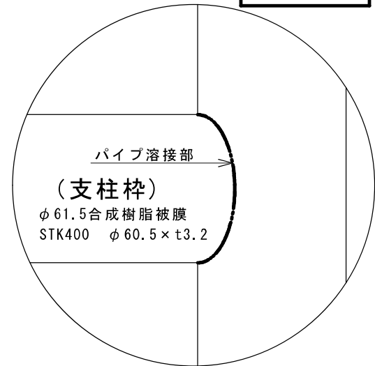
D 部詳細
