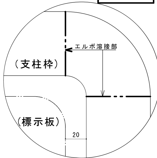
C 部詳細
