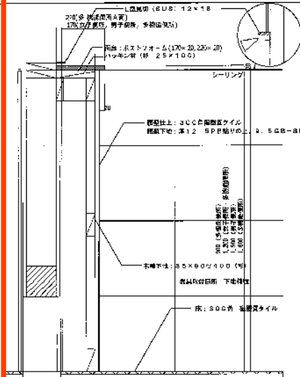
ライニング詳細図 1/10
