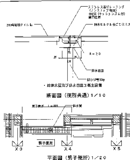
排水溝詳細図 1/10
