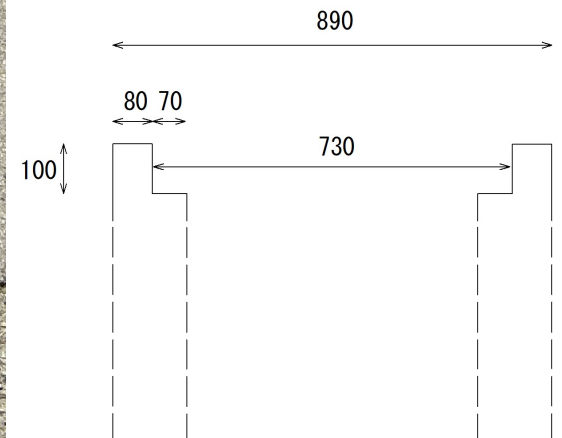
側溝イメージ図
