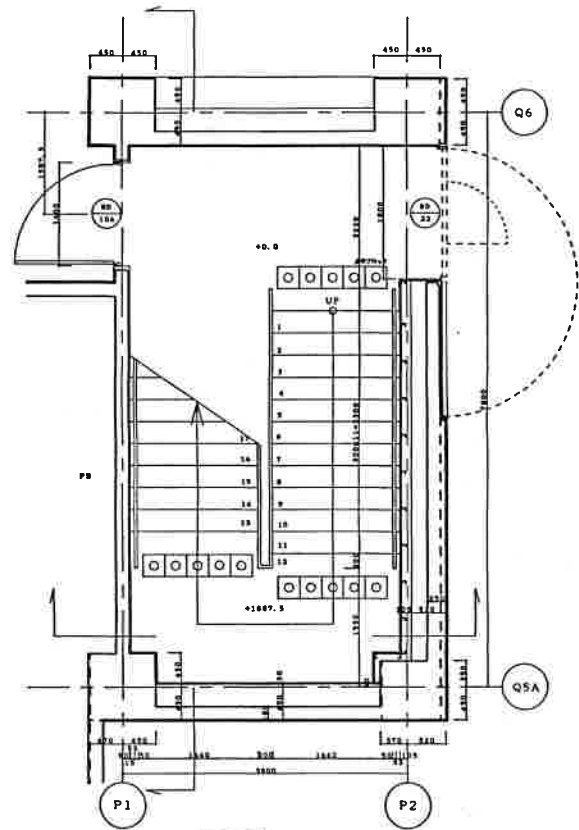
階段5 1階平面図
