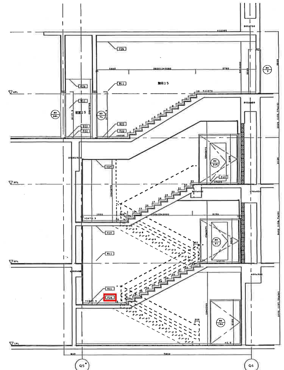
階段15 断面図2
