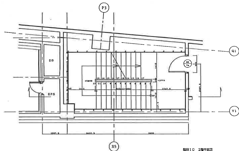
階段10 2階平面図
