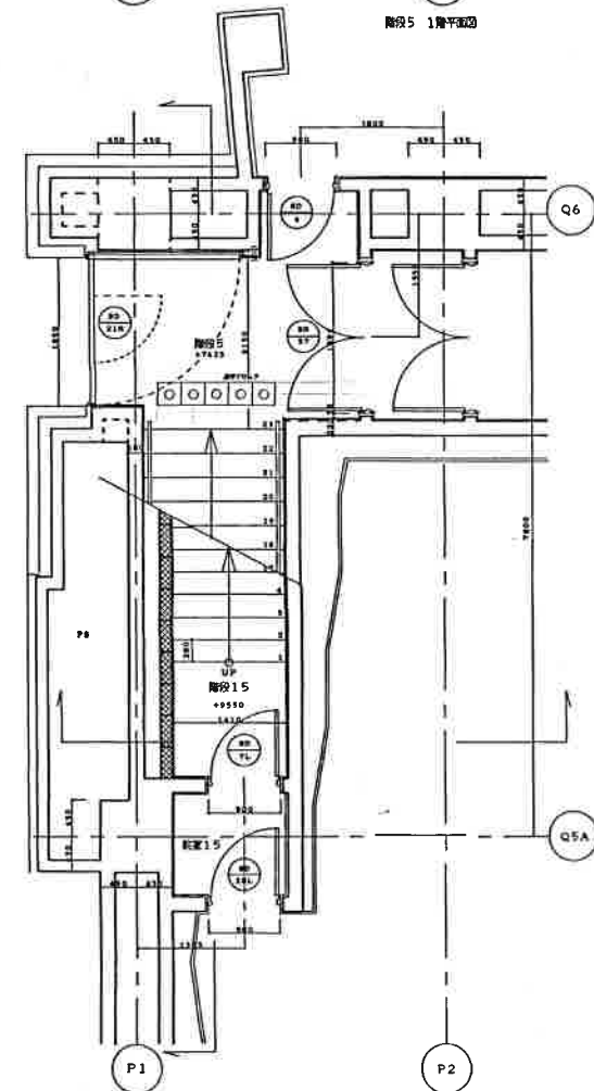
階段15 3階平面図
