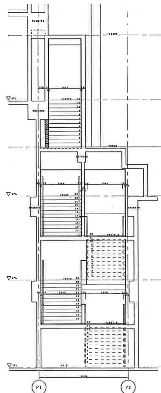
階段15 断面図1
