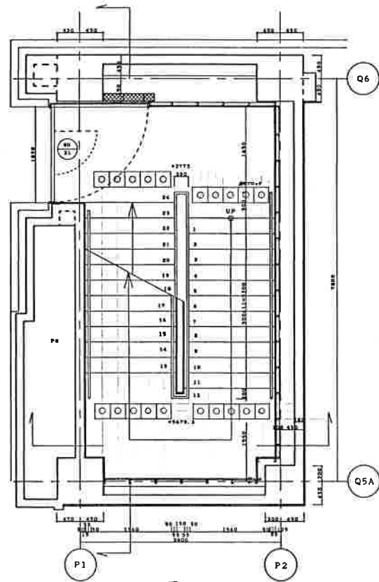
階段5 2階平面図
