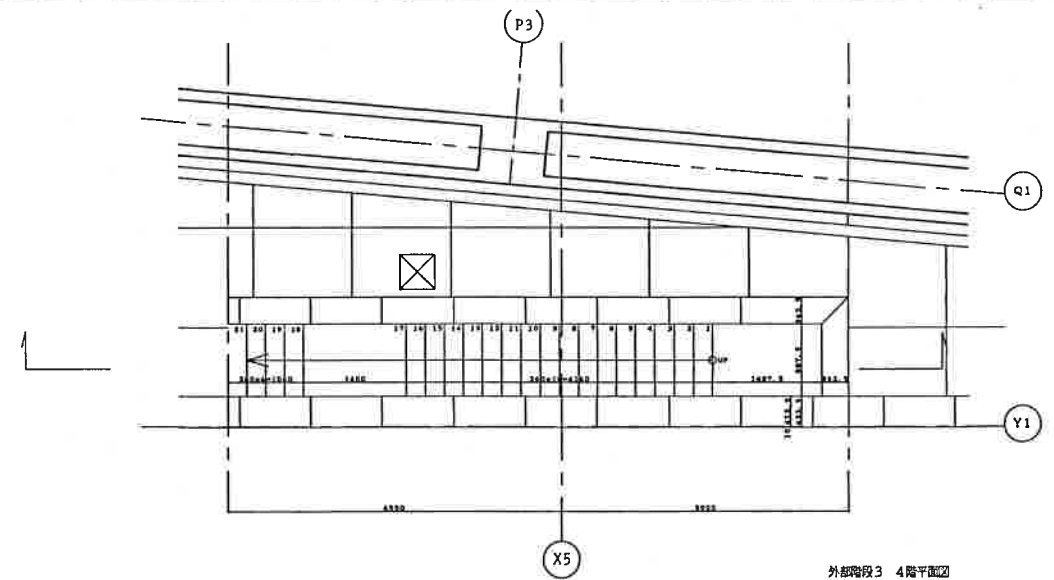
外部階段3 4階平面図
