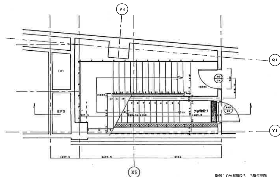
階段10外部階段3 3階平面図
