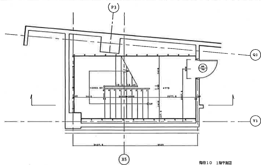
階段10 1階平面図
