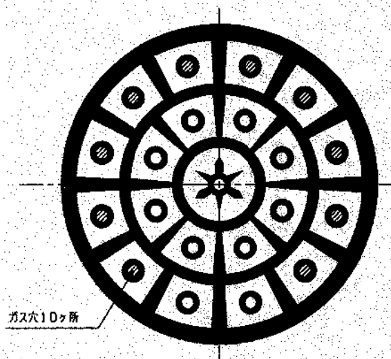
カバー平面図 (FCD AT型)
