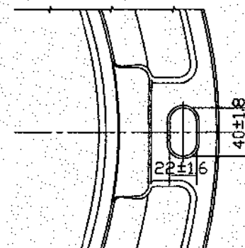
フレーム、鋳番座取付詳細図
