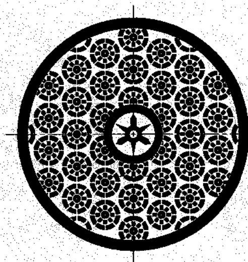
カバー平面図 (FCD BT型)
