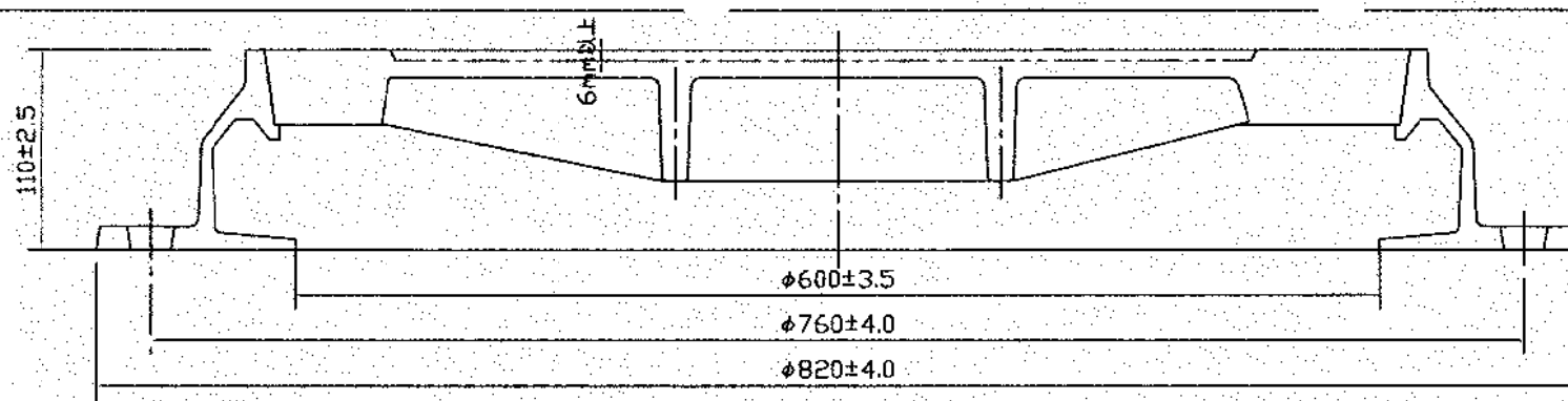
カバー、フレーム断面図
