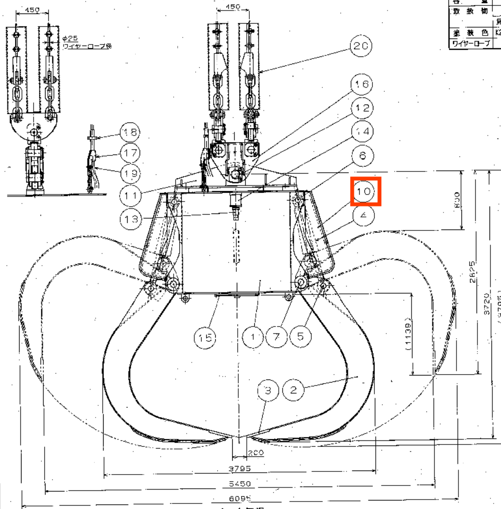
A-A矢視
