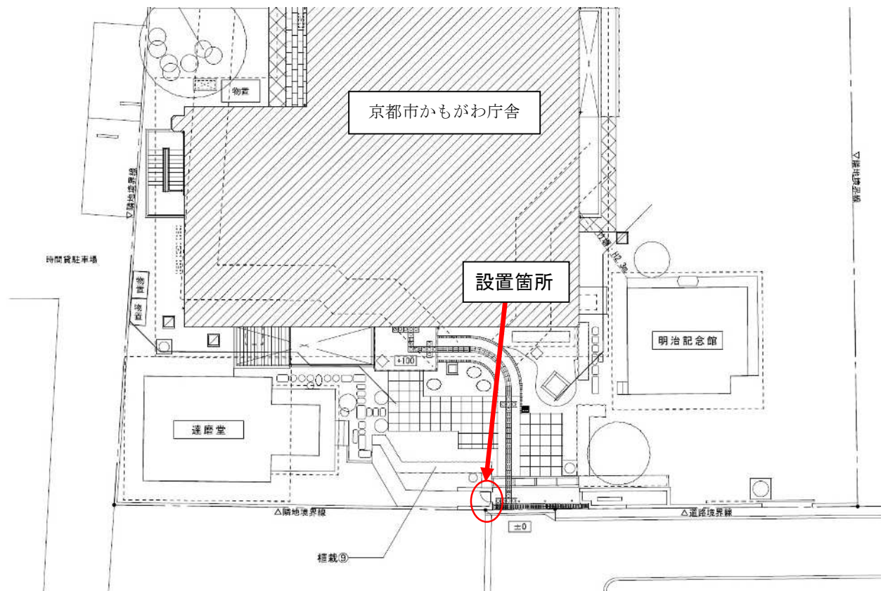
◎配置図（京都市かもがわ庁舎）
