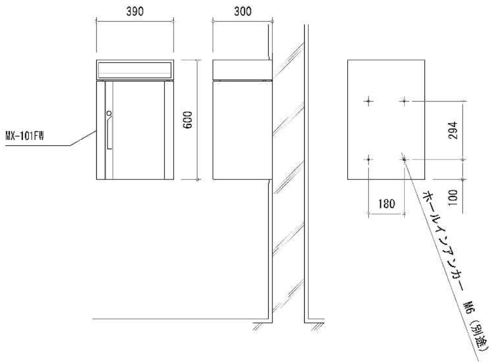
◎新設ポスト詳細図（参考）
