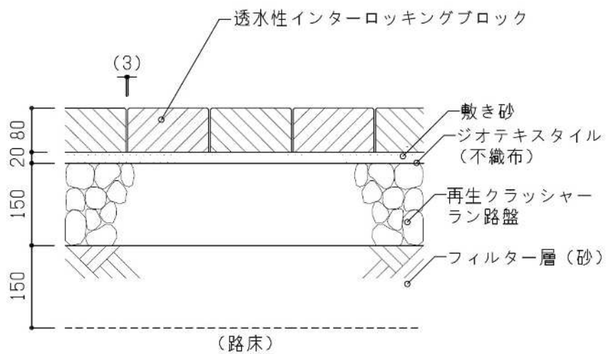
インターロッキング部分詳細図
