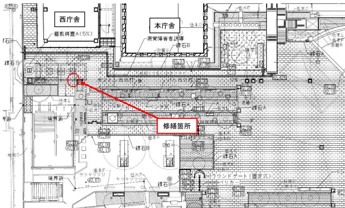
インターロッキング部分詳細図
